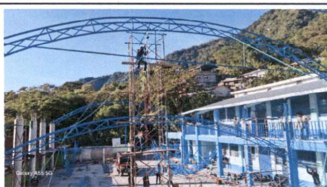
Foto 4: Instalaciones de estructura de soporte de metal por metal del patio del establecimiento.
